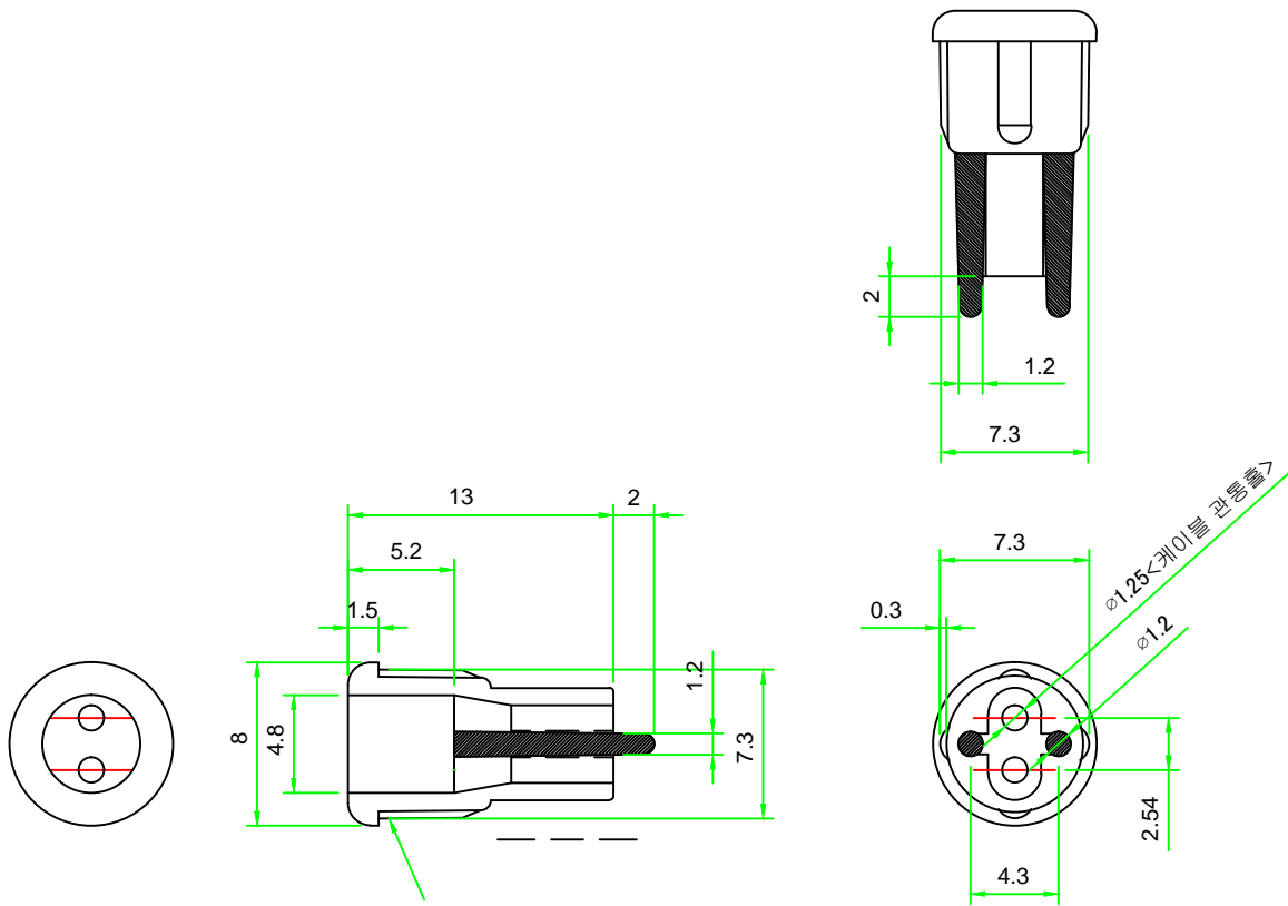
PANEL MOUNT HOLE: 7.25 (상세 치수는 샘플 실장 적용후 선택요망)
